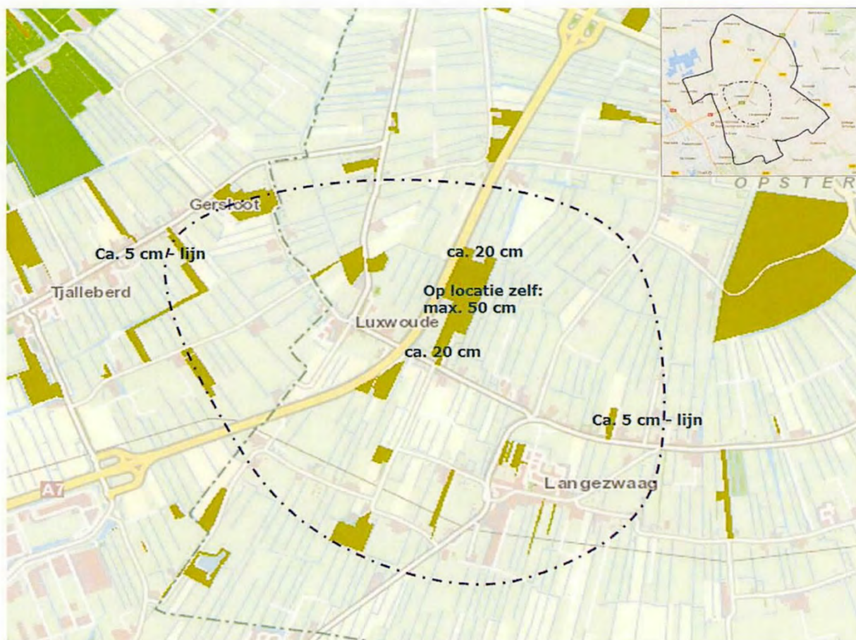
Figuur 17: globale indicatie van het gebied waar freatische grondwaterstandsverlagingen groter dan 5 cm kunnen voorkomen bij een onttrekking van 6,5 \text{ m}^3/\text{jaar}
